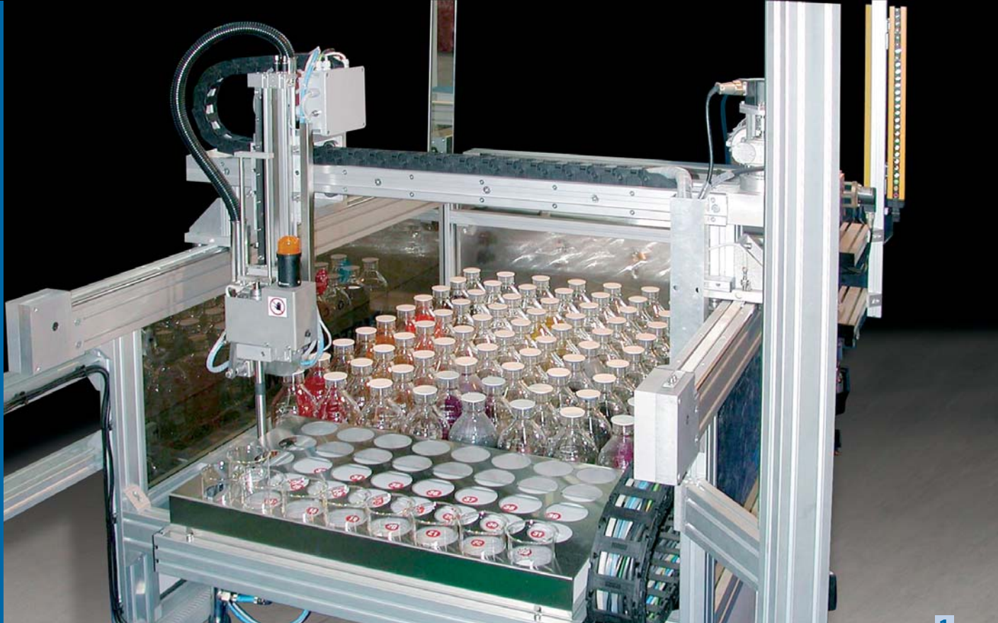
DOSATRICE AUTOMATICA DI COLORANTI E PRODOTTI CHIMICI IN SOLUZIONE CON SISTEMA VOLUMETRICO.
